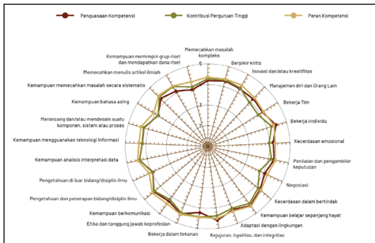
Gambar 26. Kompetensi Lulusan
