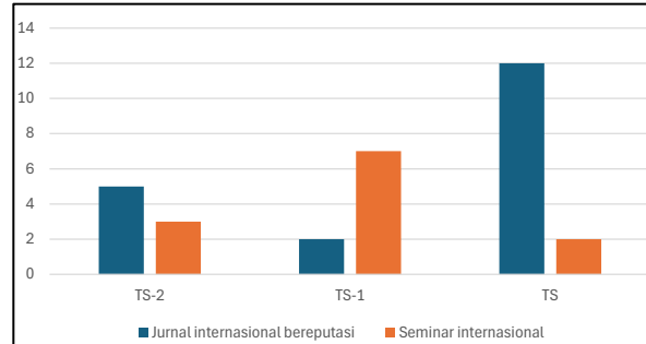
Gambar 24. Publikasi Mahasiswa
