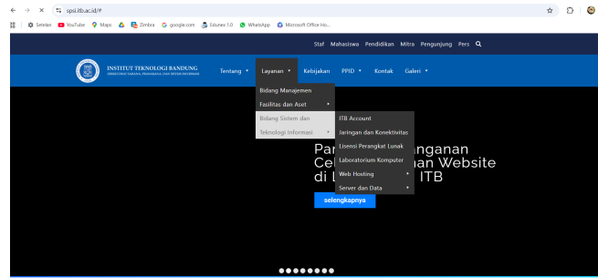
Gambar 19. Laman DTI.ITB
